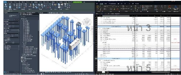
รูปที่ 12 การดำเนินการจัดกลุ่มข้อมูลโมเดลให้สอดคล้องกับ BOQ จากซอฟต์แวร์ Autodesk Revit และ Microsoft Excel
